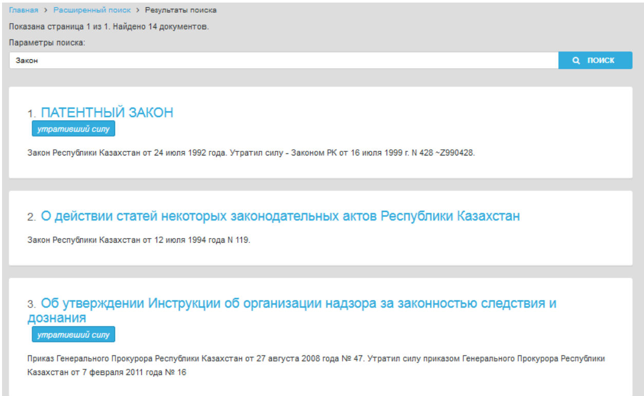
Рис. 4. Поисковая строка
